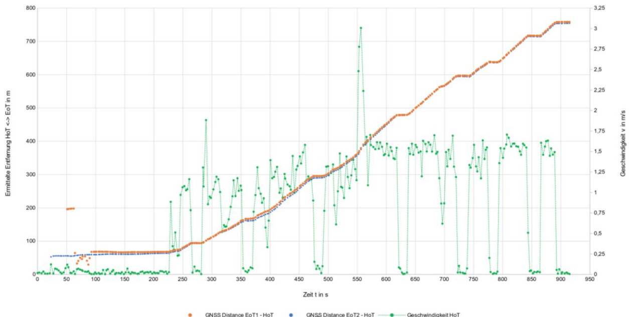
Abb. 13: Feldversuch Drehscheibe
