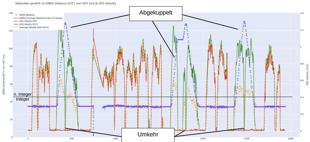
Abb. 19: Zeitabschnitt 3, DRC
