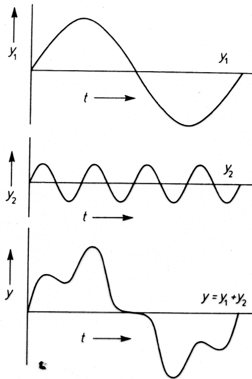
Abb. 4.5-1: Überlagerung zweier Sinus- Schwingungen y_1 + y_2 = y sehr verschiedener Frequenz
