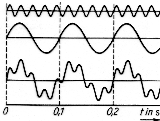
Bild 11.9. Überlagerung bei großem Frequenz- unterschied
