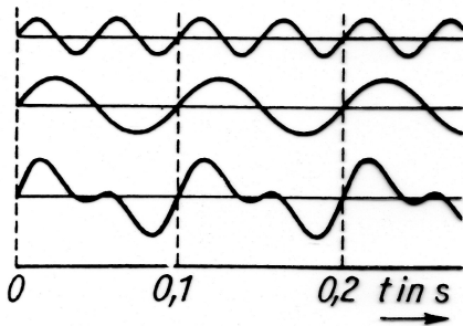
Bild 11.8. Addition zweier Schwingungen im Frequenzverhältnis 2 : 1
