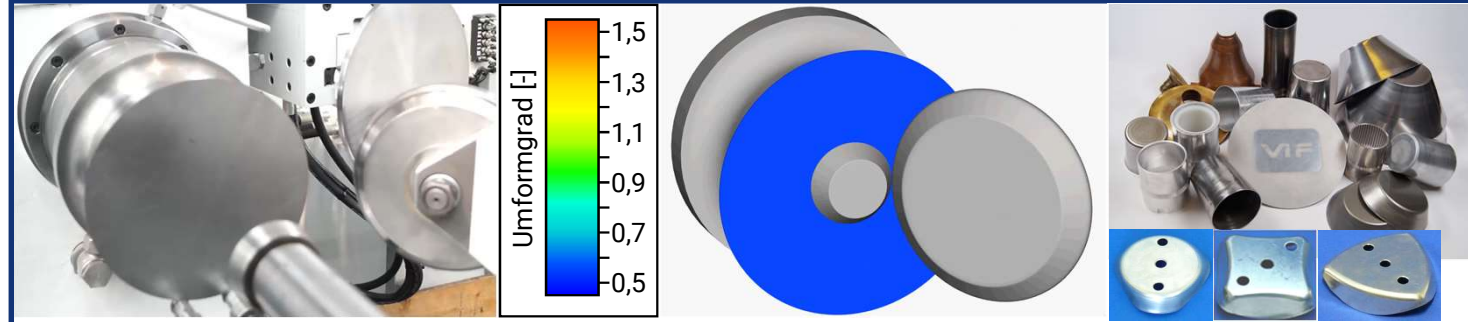
Projizierdrücken und mittels Drücken, Drückwalzen und Unrunddrücken hergestellte Bauteile
