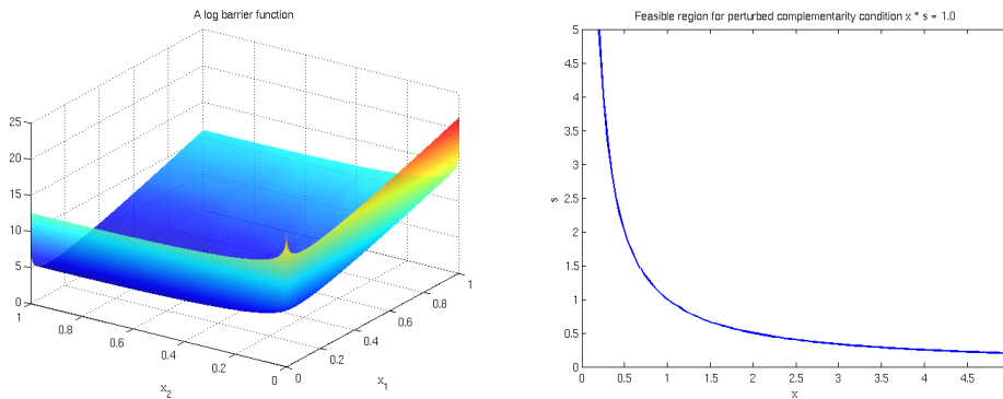
ABBILDUNG 10.1. Ein Barrierefunktional mit c = (10, 1)^\top und \tau = 1 (links) und zulässige Region bzgl. der gestörten Komplementaritätsbedingung x s = \tau (rechts).
