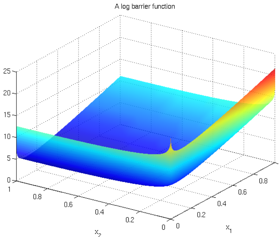
Abbildung 0.1: Graph der Barriere-Zielfunktion in (10.5) am Beispiel c = (10, 1)^\top und \tau = 1 .
