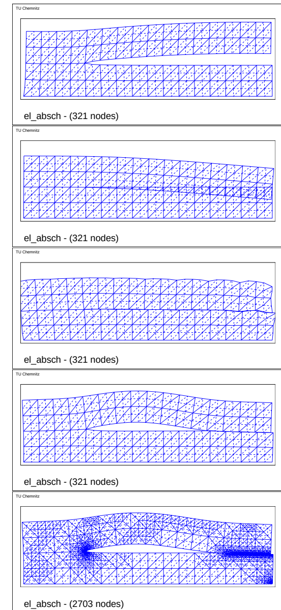
Abbildung 10: Deformierte Netze bei Rechnung in Beispiel 2
