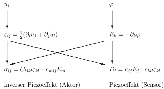
Abbildung 1: Darstellung der Abhängigkeiten bei elektromechanischen Feldgrößen
