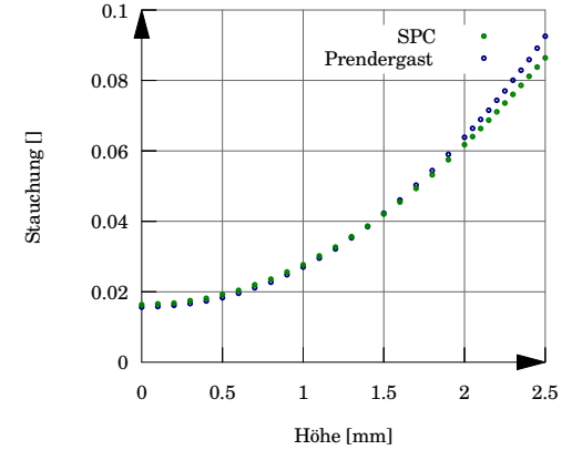
Abb. 4: Stauden im Gesenk. Darstellung des Verlaufs der axialen Stauchung über der Höhe des Knorpelzylinders (Beginn der Höhenmessung am Probenboden) zum Zeitpunkt t = 400 s. Vergleich zwischen Literaturwerten [62] und Ergebnissen von SPC-PM2AdNiMix.
