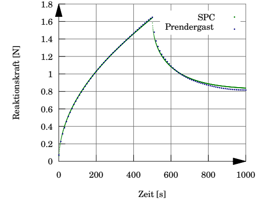
Abb. 3: Stauden im Gesenk. Darstellung der Reaktionskraft über der Zeit während der Belastungs- und Relaxationsphase. Vergleich zwischen Literaturwerten [62] und Ergebnissen von SPC-PM2AdNiMix.
