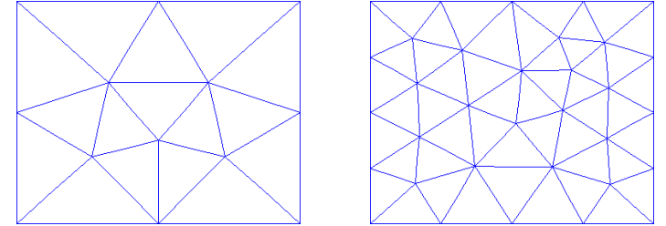
Abb. 11: Stauchen im Gesenk. Vernetzung mit 16 (links) bzw. 48 (rechts) Taylor-Hood-Dreieckelementen.
