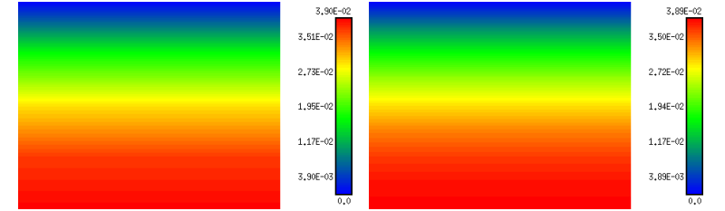
Abb. 8: Stauchen im Gesenk. Verteilung des Porenwasserdrucks (in MPa) nach jeweils 500 s. Vergleich der Ergebnisse für das Gitter mit 16 Viereckelementen (links, Gitter s. Abb. 7, p_{\max} = 0,0390 MPa) bzw. 64 Viereckelementen (rechts, Gitter s. Abb. 7, p_{\max} = 0,0389 MPa).
