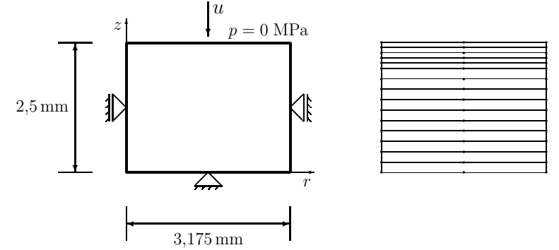
Abb. 2: Stauchen im Gesenk. Links: Geometrie und Randbedingungen des axial-symmetrischen Problems nach [62] ( u = -0,125 mm). Rechts: Originalvernetzung mit Viereckselementen nach [72].
