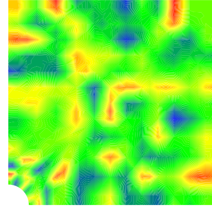
Abbildung 8: Scheibe mit Loch unter Zugbelastung in vertikaler Richtung. Darstellung von Isoflächen einer anisotropen Anfangsbelegung des durch den orthogonalen Tensor \beta im ebenen Fall repräsentierten Winkels gegenüber der horizontalen Koordinatenachse in Grad.
