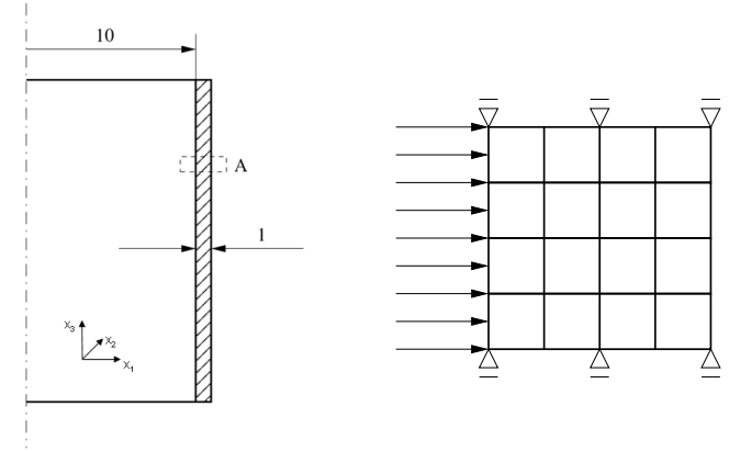
Abbildung 2: Rohr unter Innendruck. Links: Geometrie. Rechts: Ausschnitt A mit FE-Netz (16 Viereck-Elemente vom Serendipity-Typ) und Randbedingungen.
