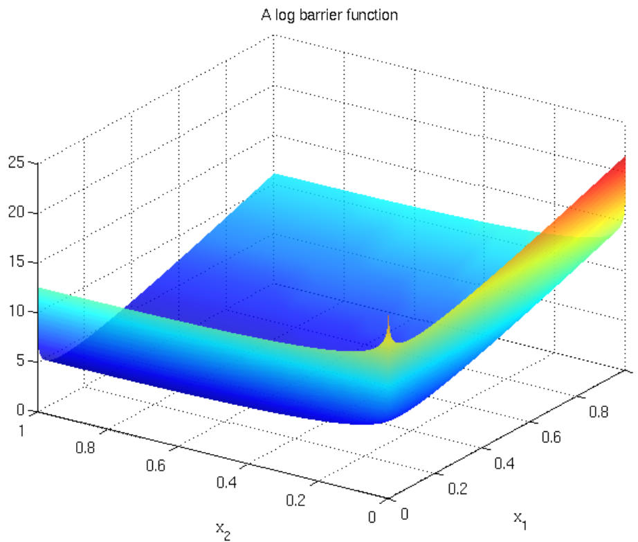
Abbildung 1: Graph der Barriere-Zielfunktion in (12.5) am Beispiel c = (10, 1)^\top und \tau = 1 .
