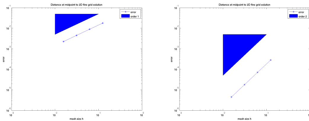
Abbildung 2: Fehler zur Feingitterlösung am Mittelpunkt des Einheitsquadrates für obige Approximationen 1. Ordnung (links) bzw. 2. Ordnung (rechts) der Robin-Randbedingungen.
