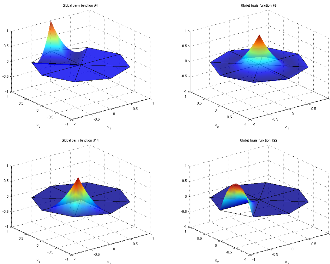
Abbildung 2: Einige globale Formfunktionen für einen FE-Raum aus global stetigen \mathbb{P}_2 -Elementen
