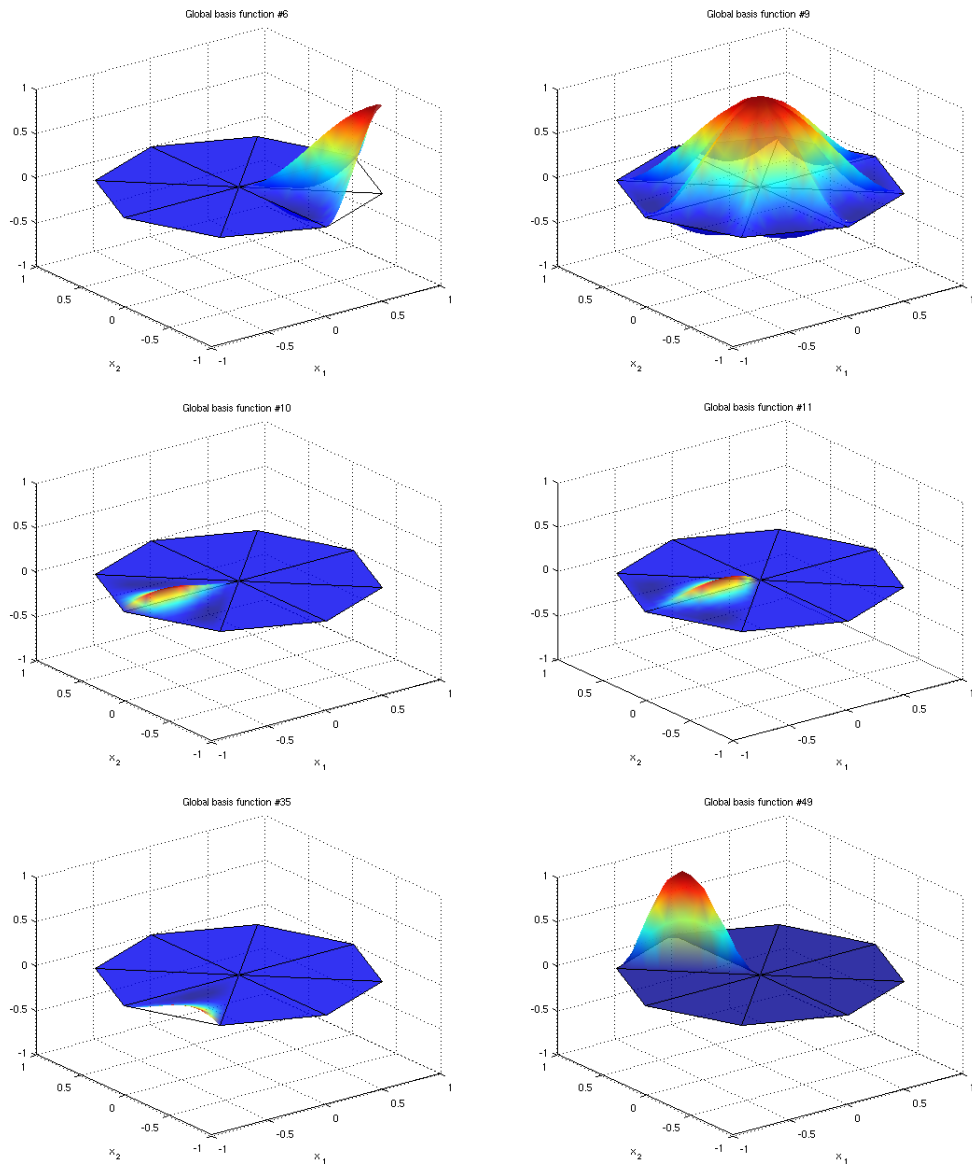
Abbildung 3: Einige globale Formfunktionen für einen FE-Raum aus global stetigen kubischen Hermite-Elementen
