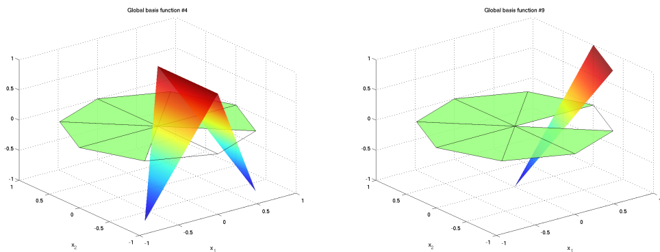
Abbildung 4: Einige globale Formfunktionen für einen FE-Raum aus (linearen) Crouzeix-Raviart-Elementen
