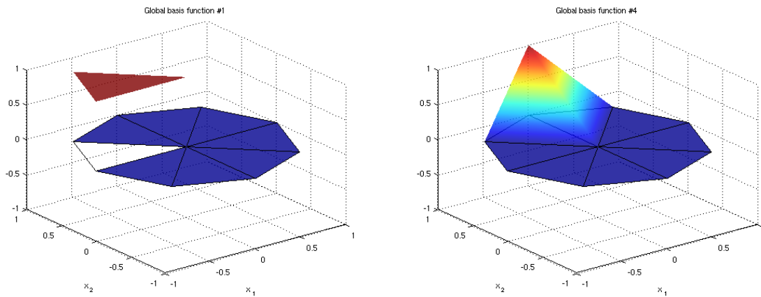
Abbildung 1: Einige globale Formfunktionen für einen FE-Raum aus \mathbb{P}_0 - und global stetigen \mathbb{P}_1 -Elementen
