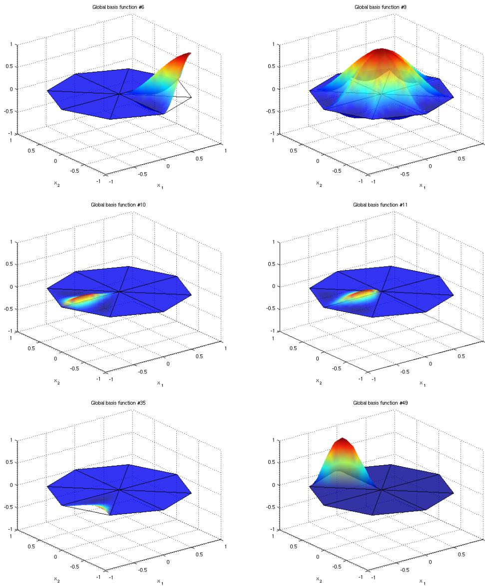
Abbildung 3: Einige globale Formfunktionen für kubische Hermite-Elemente
