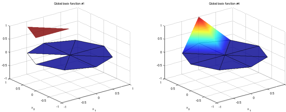
Abbildung 1: Einige globale Formfunktionen für \mathbb{P}_0 - und \mathbb{P}_1 -Elemente
