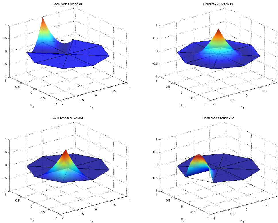
Abbildung 2: Einige globale Formfunktionen für \mathbb{P}_2 -Elemente
